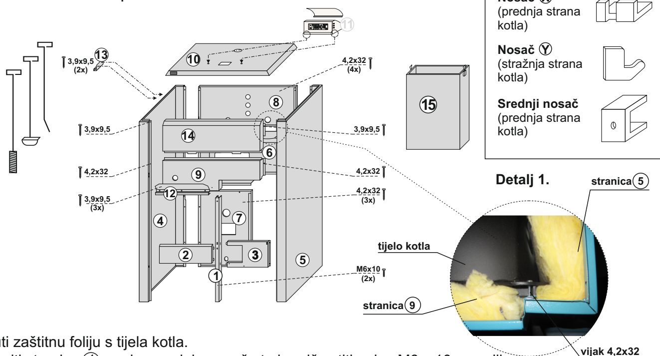
Slika 2. Montaža oplata na kotao
