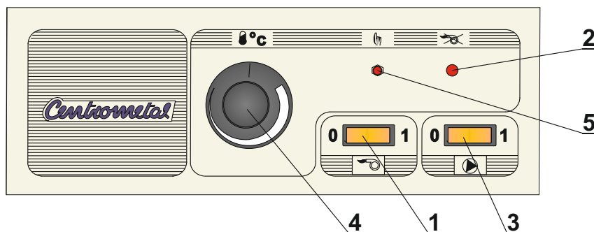
Slika 5. Osnovna kotlovska regulacija
