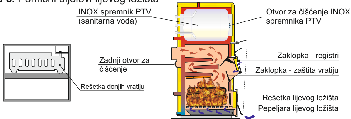
Slika 7. Pomični dijelovi desnog ložišta
