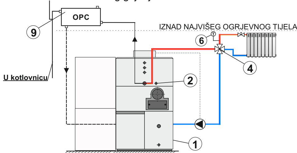
Shema 3b. Primjer kada prema EN 303-5 nije potrebna ugradnja akumulacijskog spremnika u sustav centralnog grijanja
