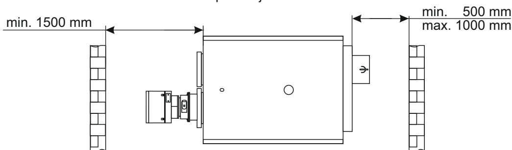
Slika 4a. Minimalni razmak od zidova prostorije
