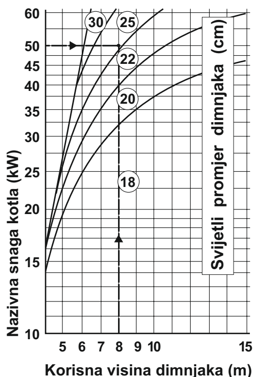
Slika 4. Dimenzioniranje dimnjaka za kotlove CentroPlus-B
