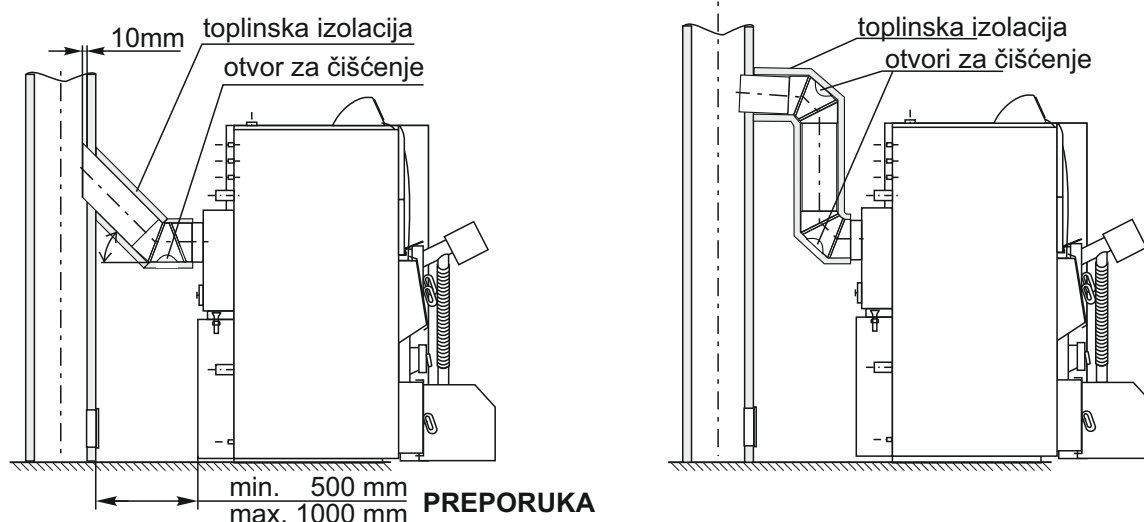
Slika 3. Mogući načini priključenja kotlova CentroPlus-B na dimnjak
