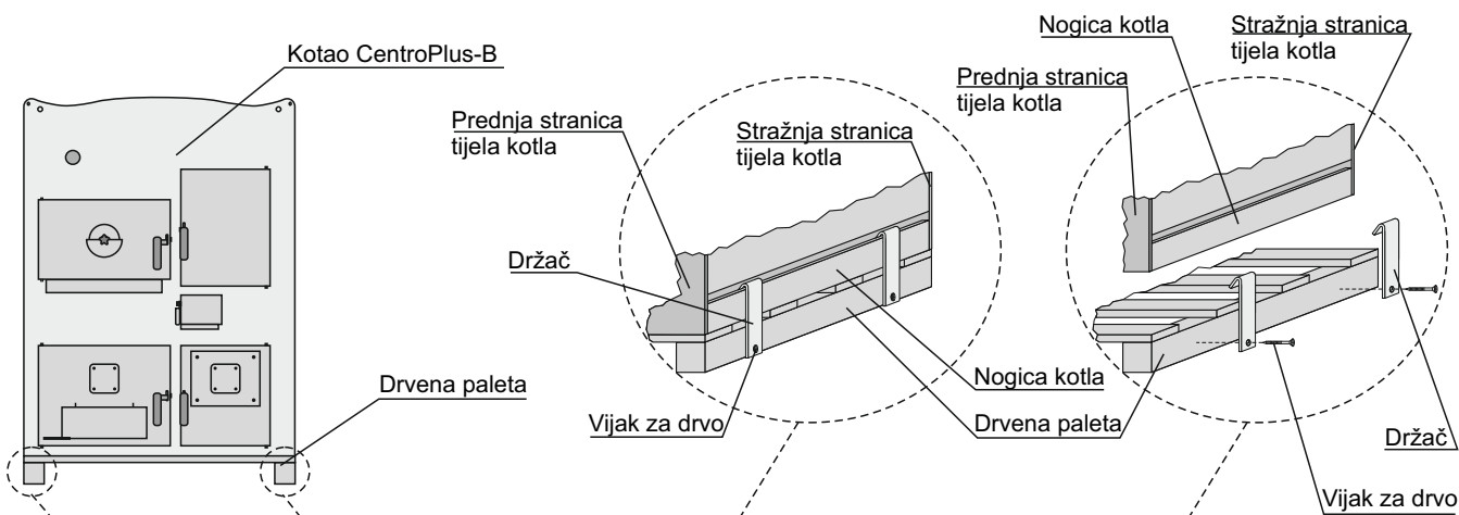
Slika 1. - Skidanje kotla sa drvene palete
