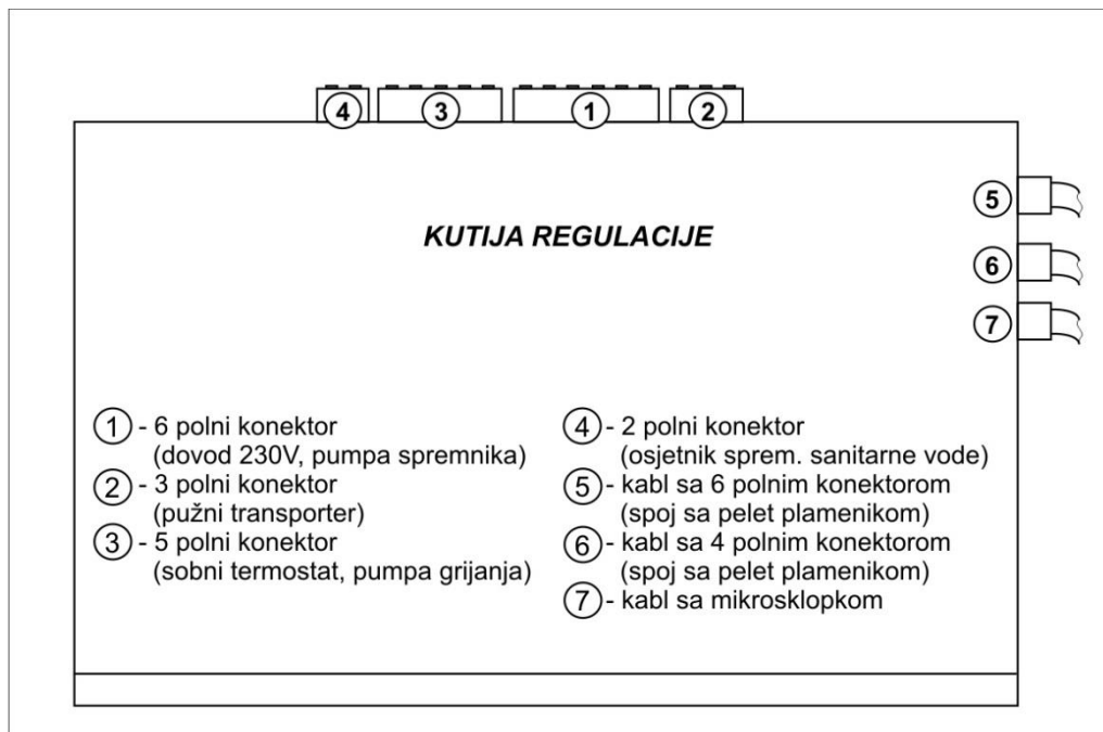
Slika: Prikaz konektora na kutiji regulacije
