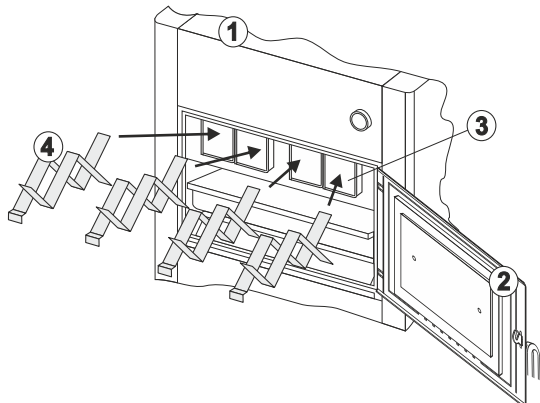
Slika 11. Prikaz ugradnje turbulatora
