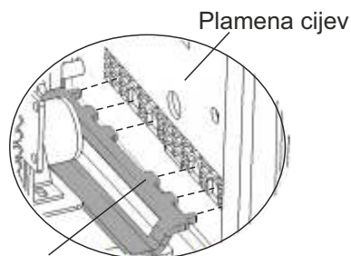
Zaštita rupe plamene cijevi
