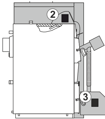
2. Regulacija 3. Plamenik
