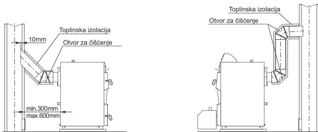
Slika 7. Mogući načini priključenja kotla EKO-CK (B) P + Cm Pelet-set na dimnjak
