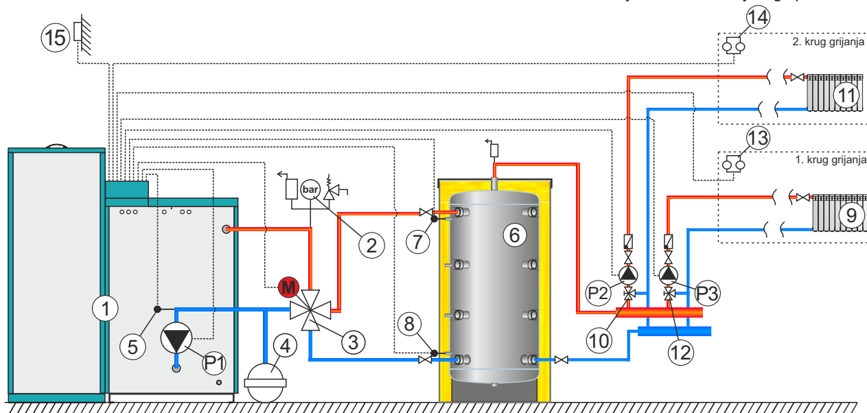
Shema 14. Konfiguracija AKU--IKG x2
