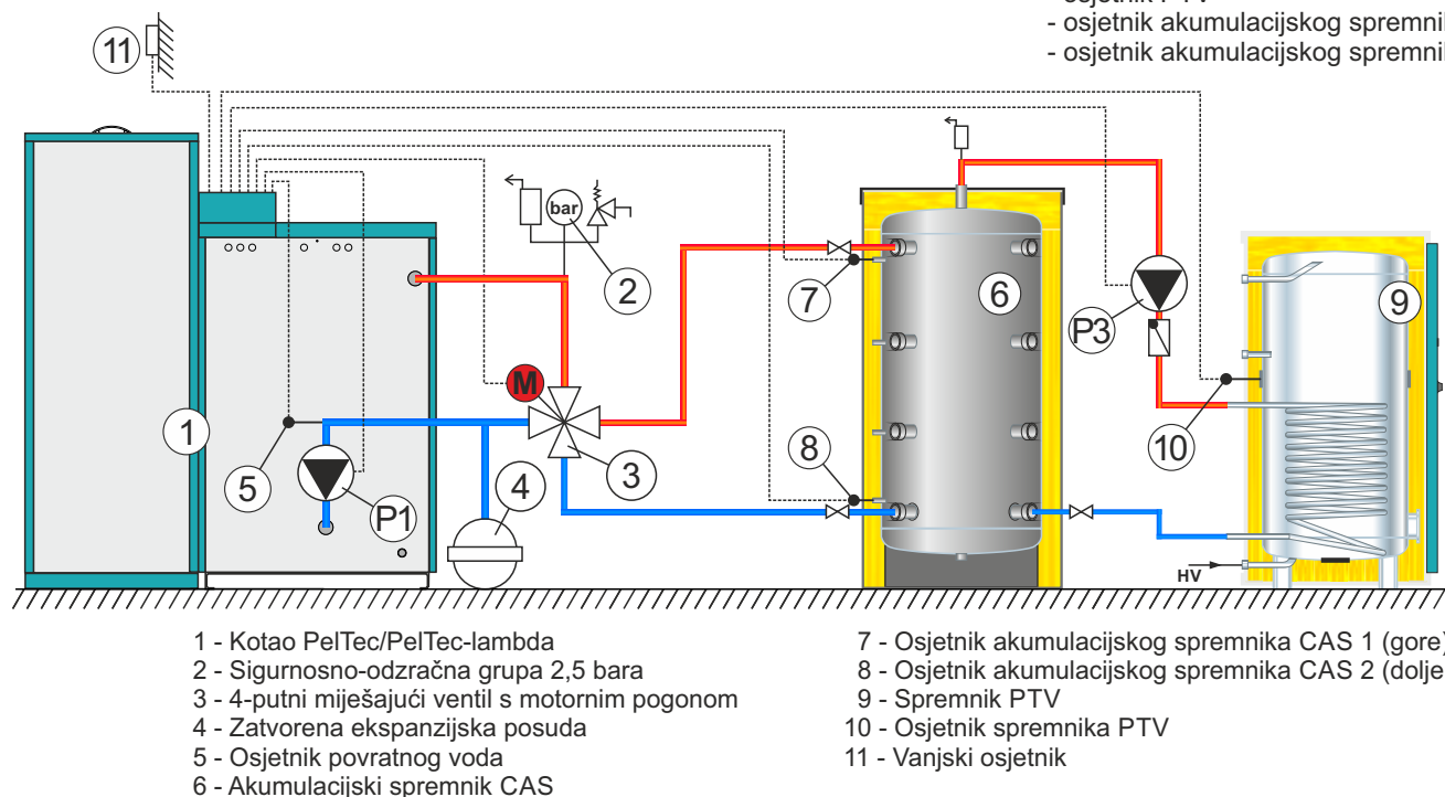
Shema 8. Konfiguracija AKU -- PTV
