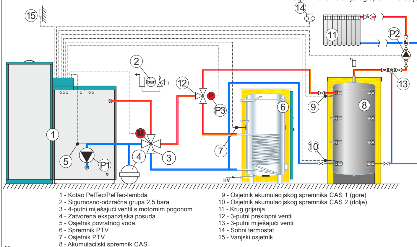
Shema 7. Konfiguracija PTV || AKU -- IKG
