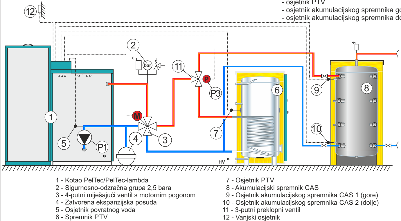
Shema 5. Konfiguracija PTV || AKU
