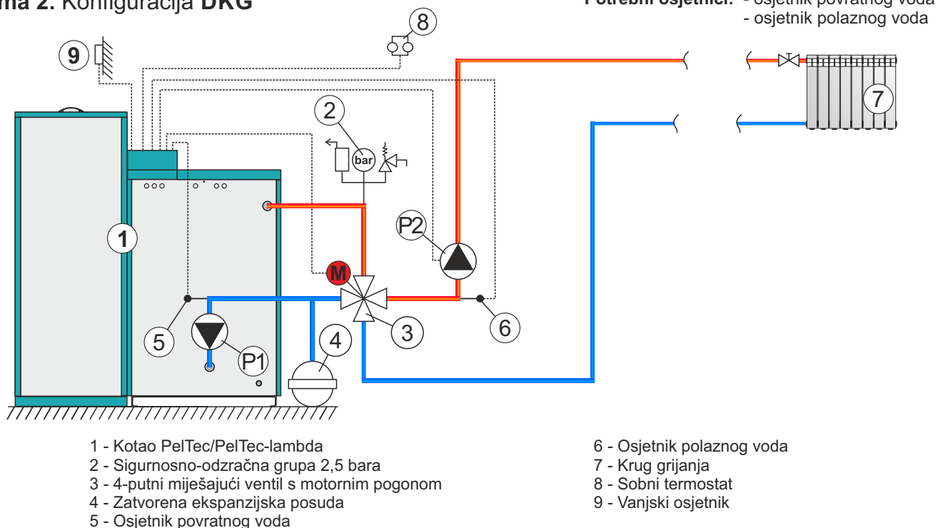
Shema 2. Konfiguracija DKG
