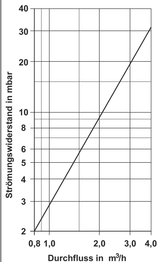
Abbildung 1. Strömungswiderstand
