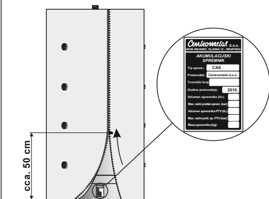
Slika 2. Položaj natpisne pločice na akumulacijskom spremniku
