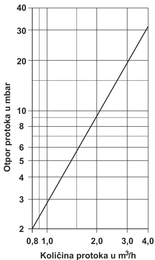
Slika 1. Otpor protoka
