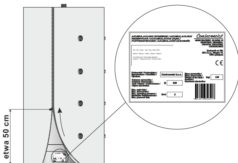
Abbildung 2. Position des Aufklebers auf dem Pufferspeicher
