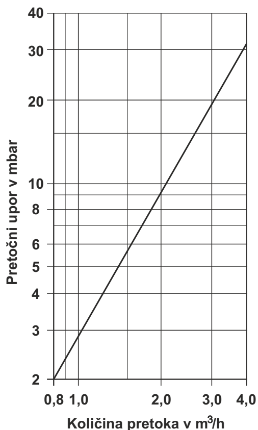
Slika 1. Pretočni upor
